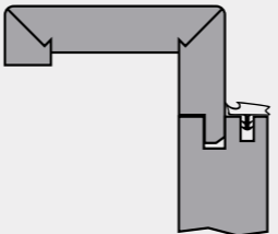
4 ZARGE MIT KLEINER RUNDKANTE FRAME WITH SMALL ROUNDED EDGE
