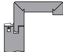
ZARGE MIT KLEINER RUNDKANTE, 60 MM BEKLEIDUNG FRAME WITH SMALL ROUNDED EDGE, 60 MM CASING
