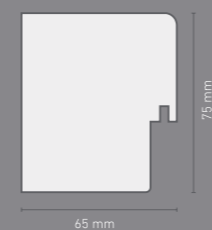
Wandprofil Wall edge
