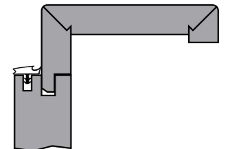
ZARGE MIT KLEINER RUNDKANTE, 100 MM BEKLEIDUNG FRAME WITH SMALL ROUNDED EDGE, 100 MM CASING
