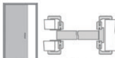
Schiebetür in der Wand laufend (GARANT: links öffnend) (DIN 107: rechts schließend)
