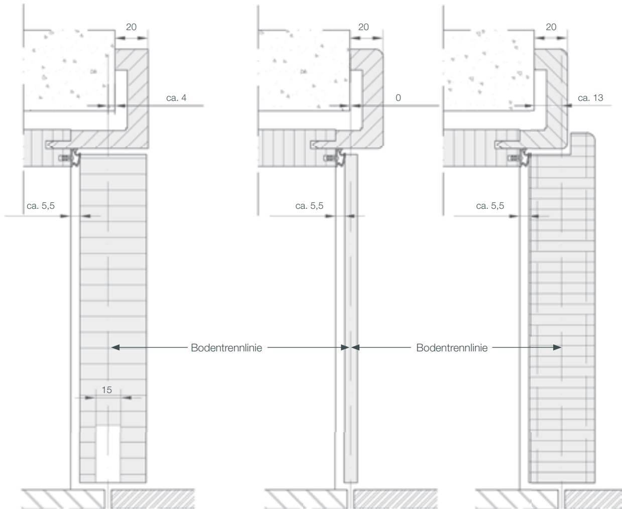
Türblatt ca. 40 mm stumpf, mit und ohne Bodendichtung
