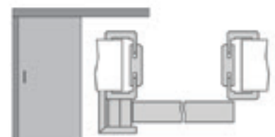
Schiebetür vor der Wand laufend (GARANT: rechts öffnend) (DIN 107: links schließend)
