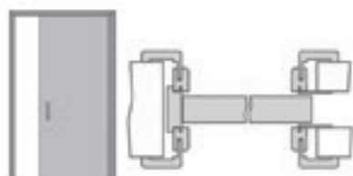
Schiebetür in der Wand laufend (GARANT: rechts öffnend) (DIN 107: links schließend)
