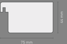
Aufbau Blendrahmen Blind frame construction
