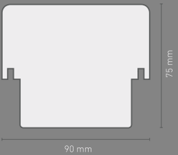
Kämpfer / Pfosten Traverse / Pole
