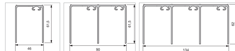
solido MS Führungsschiene
