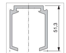
solido MS-H Führungsschiene
