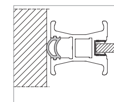
Anschlagdichtung
