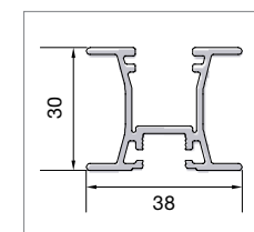
Griffprofil BAL
